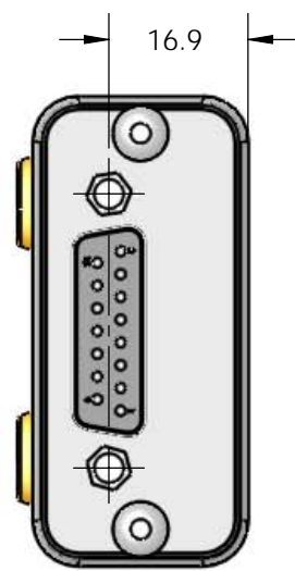
DB-15 INPUT
